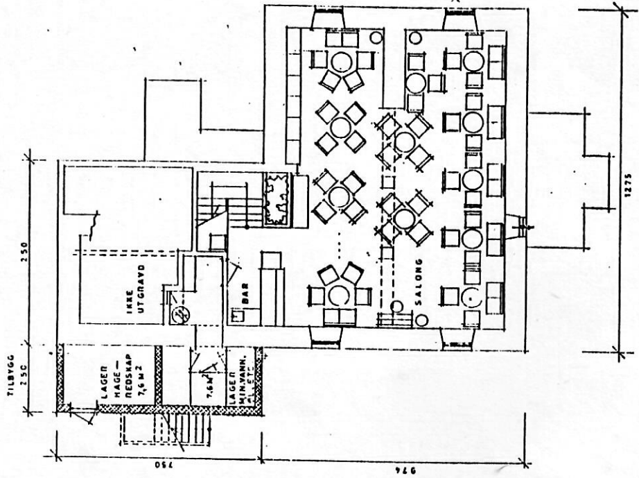
PLAN KJELLER
