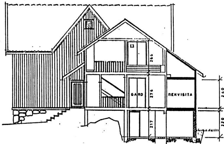
SNITT
